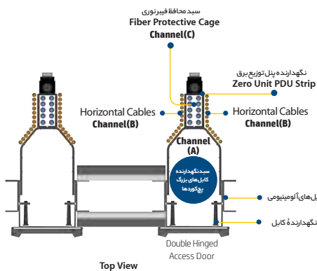
تصویر از نمای بالای رک Open Frame
